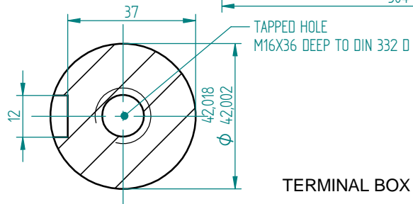
Przekrój A-A 1:1
